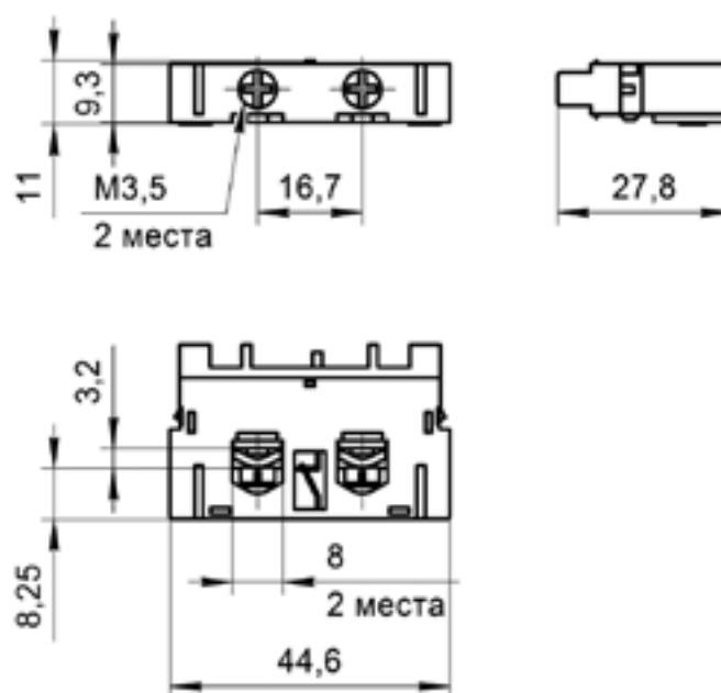
Контакт вспомогательный АВАН-ВКП
