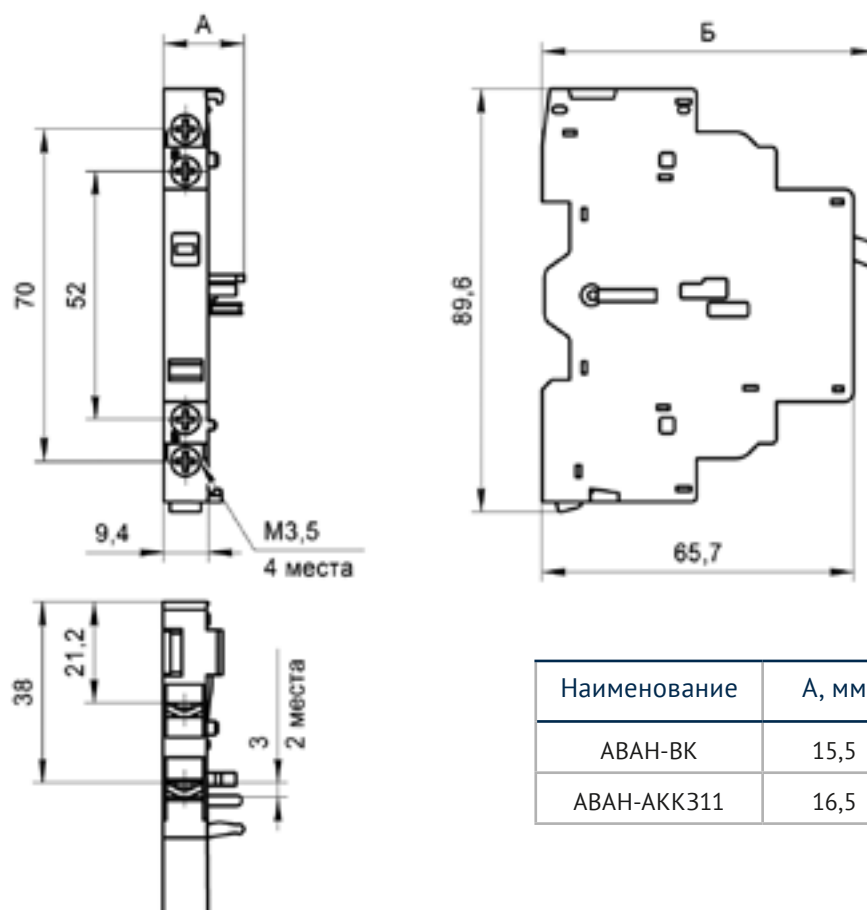
Контакт вспомогательный АВАН-ВК и контакт сигнализации короткого замыкания АВАН-АККЗ
